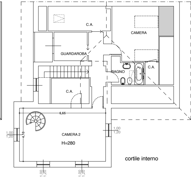
PIANO SOTTOTETTO
