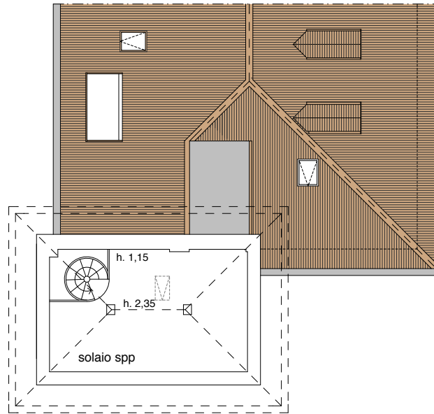
PIANO SOLAIO
